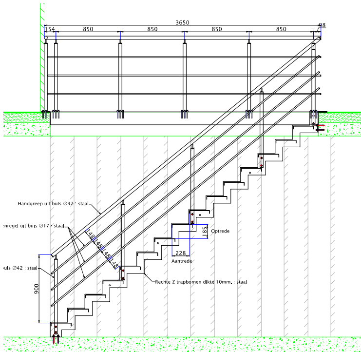
Autocad-tekening van uw project Dessin AutoCAD de votre projet
