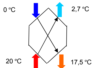
Schematische weergave wisselaar
